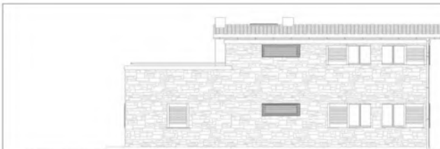
prospetto NORD
