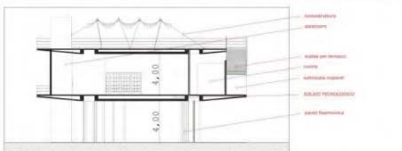
sezione a-a'
