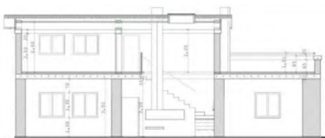
sezione P/1
